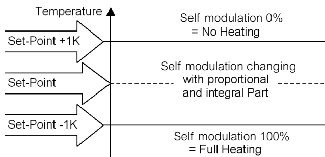
Temperaturområde för självmodulering, cykeltid 42 min.
